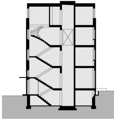
Schnitt A-A
